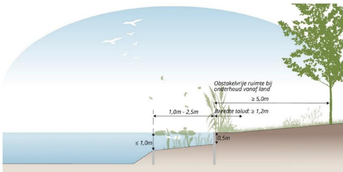
Figuur 4.4. Voorbeeld: NVO: Onderwaterbanket met verdediging zonder bovenwaterbeschoeiing (Bron: TAUW).
