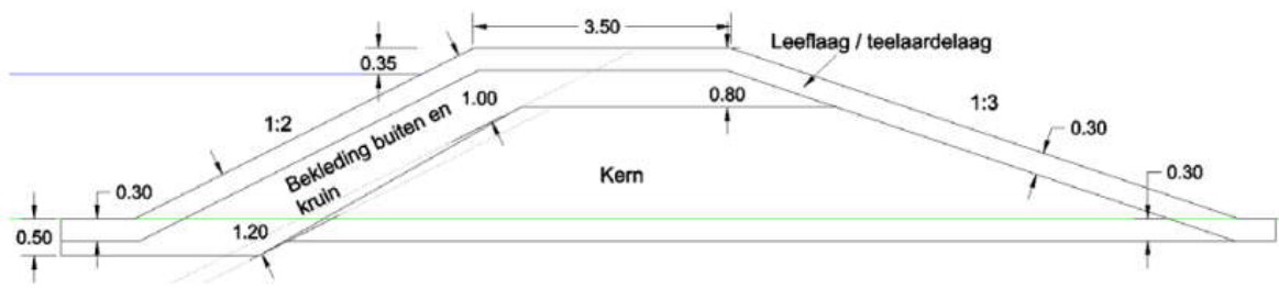
Figuur 3-2: Opbouw dam (schetsmatig)
