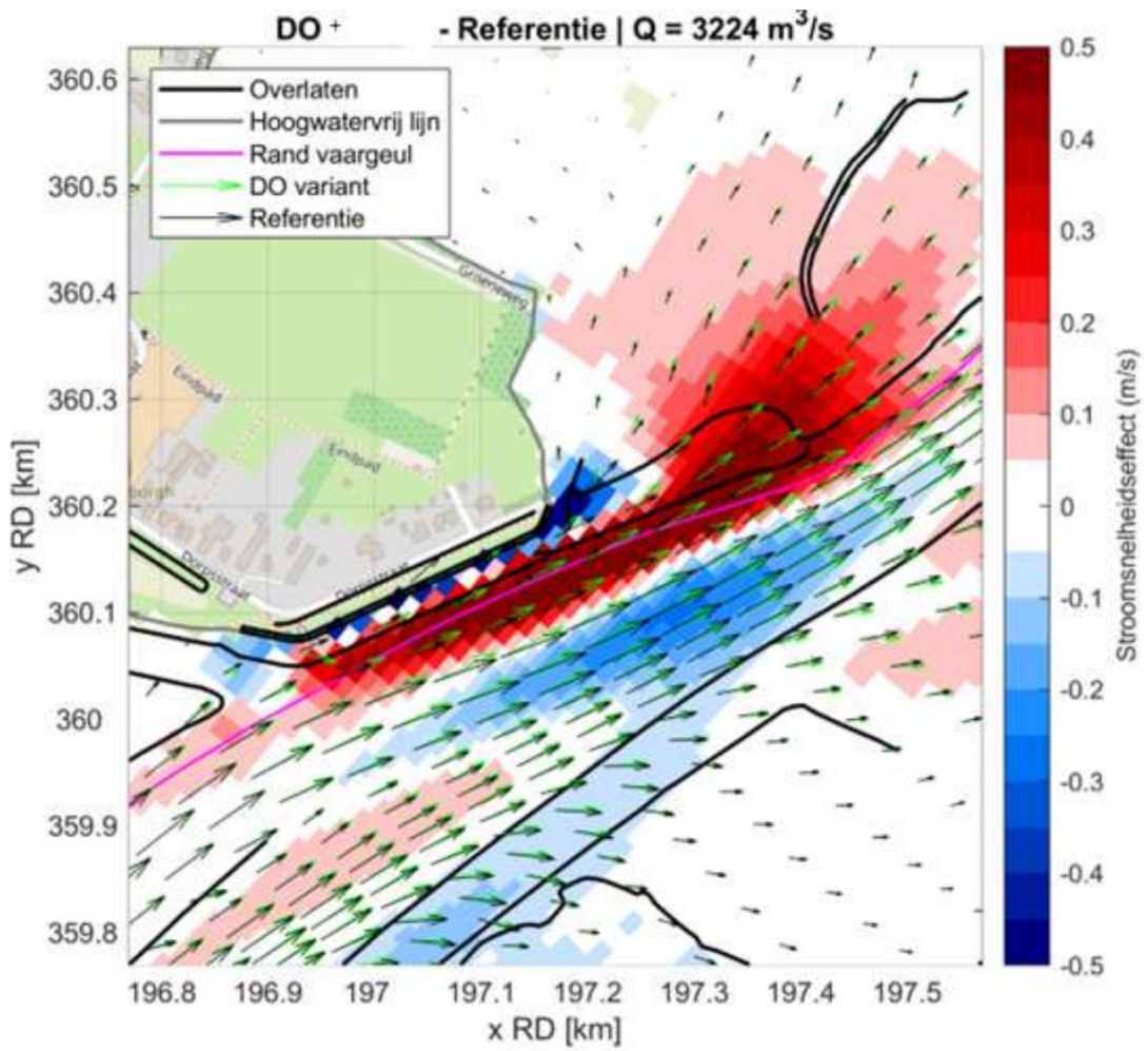
Fig. E.16: Detail van het stroomsnelheidseffect ten gevolge van het DO+ rondom de projectlocatie bij een afvoer van 3224 m 3 /s. Een rode kleur betekent een verhoging van de stroomsnelheid door het DO+.
