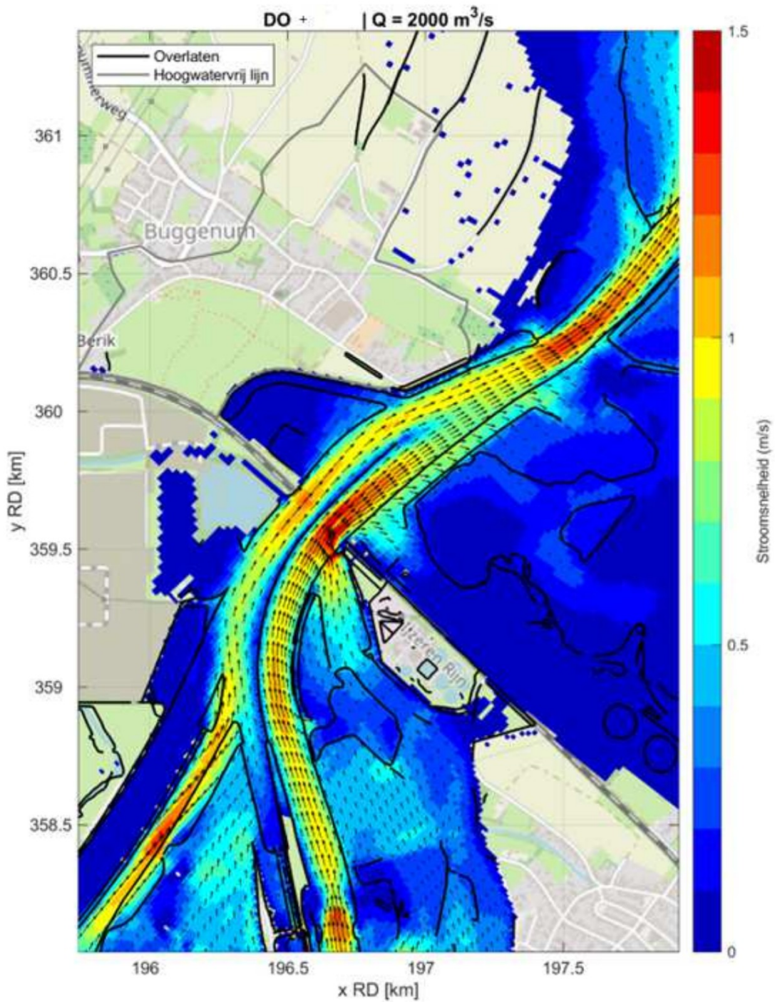
Fig. E.10: Stroomsnelheden in het geval van het DO+ rondom de projectlocatie bij een afvoer van 2000 m 3 /s.
