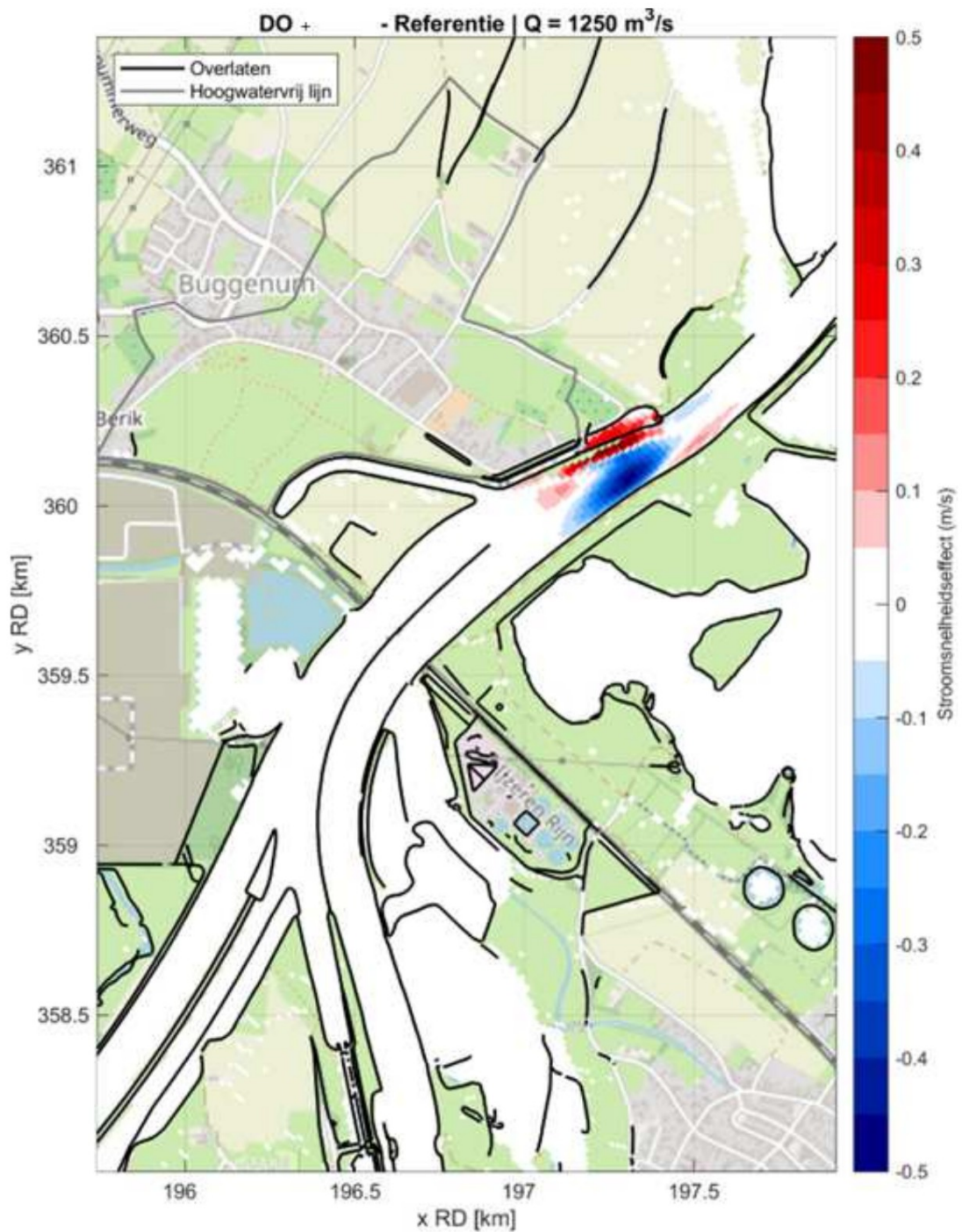
Fig. E.3: Stroomsnelheidseffect ten gevolge van de DO + rondom de projectlocatie bij een afvoer van 1250 m 3 /s. Een rode kleur betekent een verhoging van de stroomsnelheid door de DO +.
