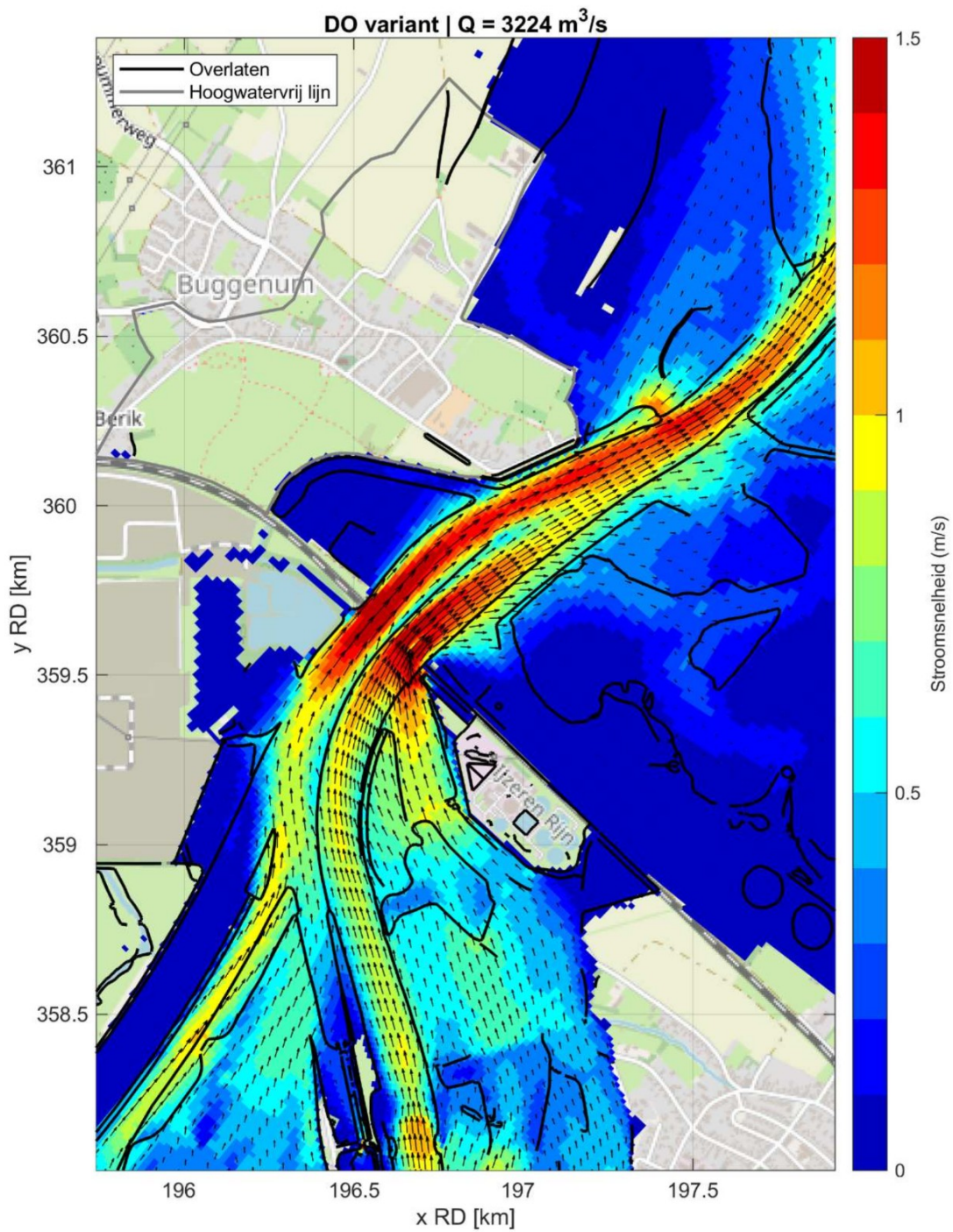
Fig. E.14: Stroomsnelheden in het geval van het DO+ rondom de projectlocatie bij een afvoer van 3224 m 3 /s.
