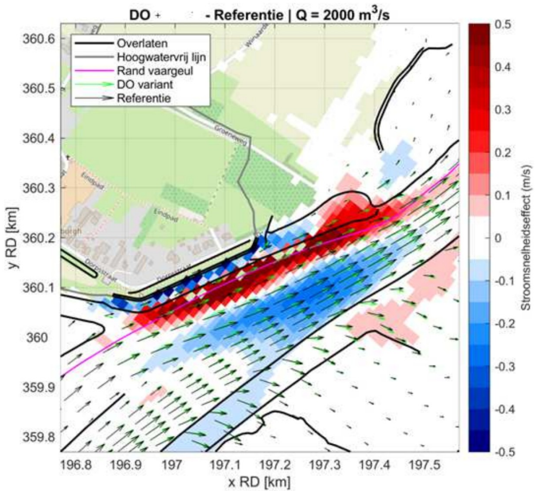
Fig. E.12: Detail van het stroomsnelheidseffect ten gevolge van het DO+ rondom de projectlocatie bij een afvoer van 2000 m 3 /s. Een rode kleur betekent een verhoging van de stroomsnelheid door het DO+.
