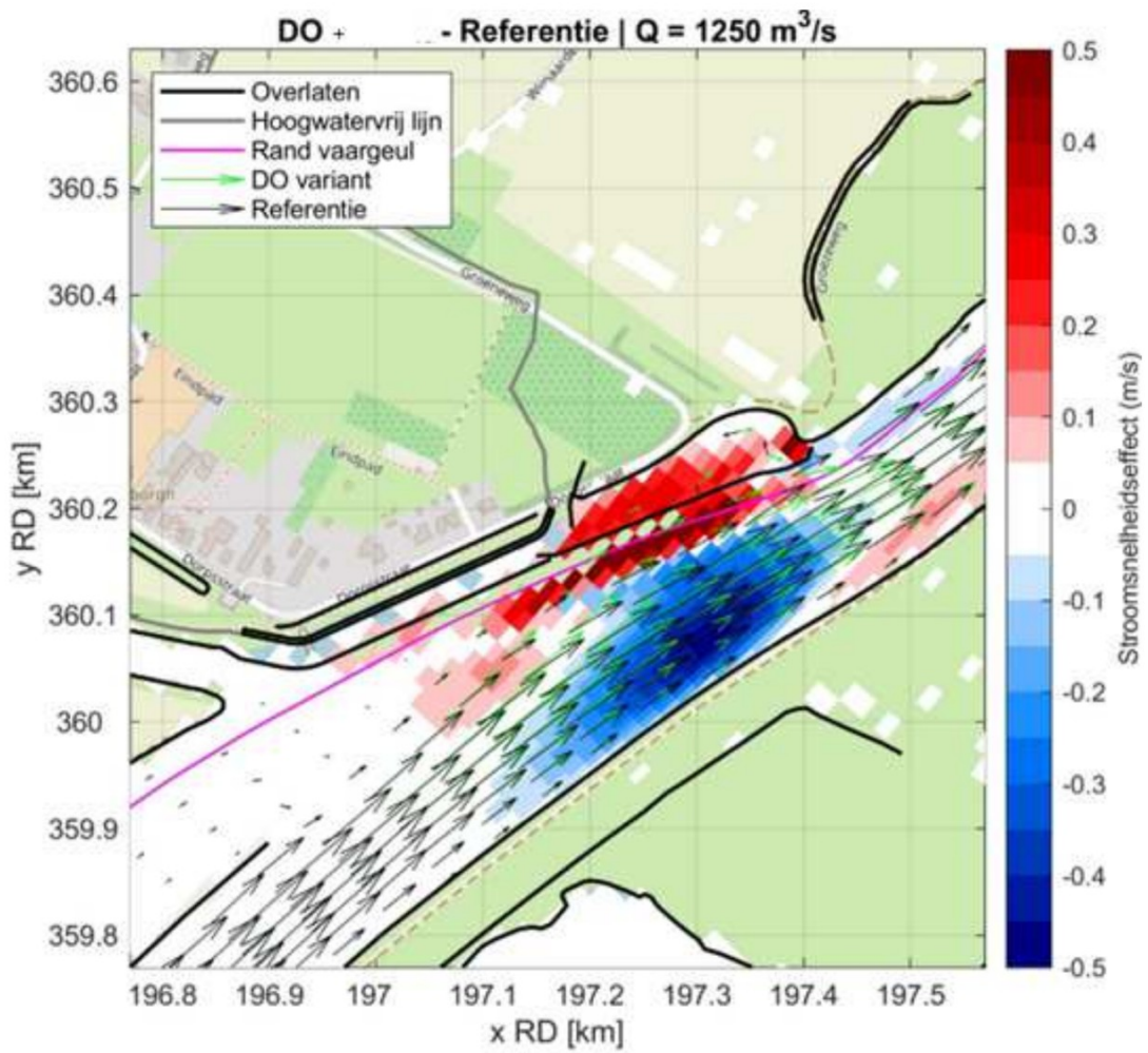
Fig. E.4: Detail van het stroomsnelheidseffect ten gevolge van het DO+ rondom de projectlocatie bij een afvoer van 1250 m 3 /s. Een rode kleur betekent een verhoging van de stroomsnelheid door de DO+.
