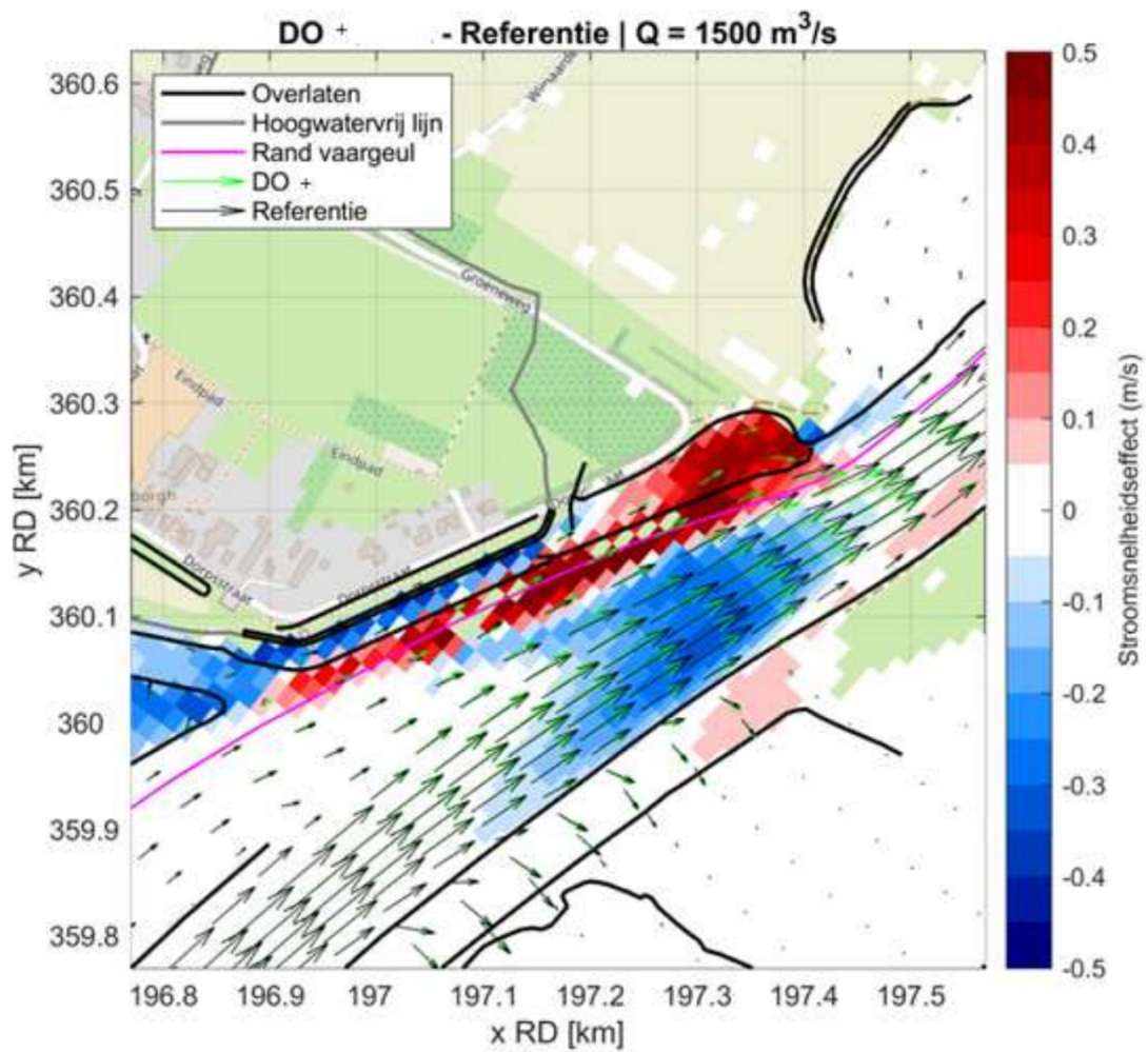
Fig. E.8: Detail van het stroomsnelheidseffect ten gevolge van het DO + rondom de projectlocatie bij een afvoer van 1500 m 3 /s. Een rode kleur betekent een verhoging van de stroomsnelheid door het DO +.
