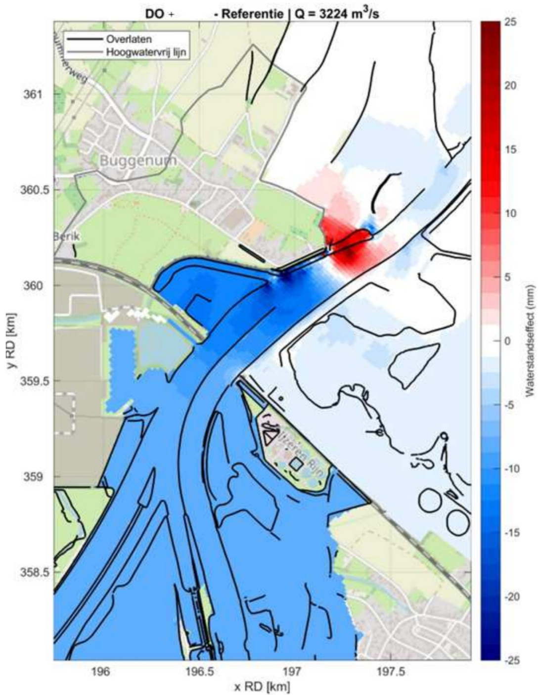
Fig. D.3: Waterstandseffect ten gevolge van het DO+ rondom de projectlocatie bij een afvoer van 3224 m 3 /s. Een rode kleur betekent een verhoging van de waterstand door het DO+.
