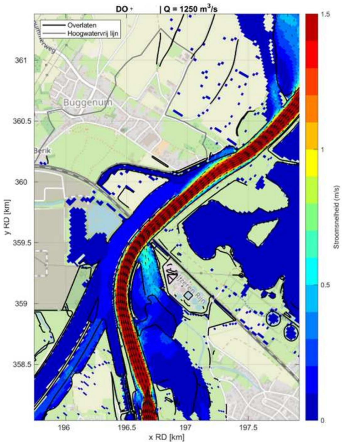
Fig. E.2: Stroomsnelheden in het geval van de DO+ rondom de projectlocatie bij een afvoer van 1250 m 3 /s.
