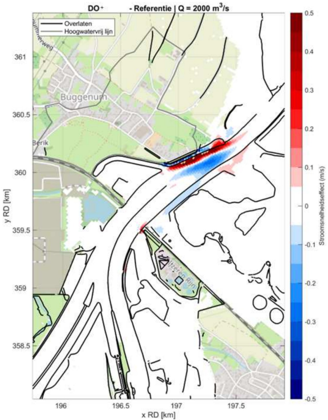
Fig. E.11: Stroomsnelheidseffect ten gevolge van het DO+ rondom de projectlocatie bij een afvoer van 2000 m 3 /s. Een rode kleur betekent een verhoging van de stroomsnelheid door de DO+.
