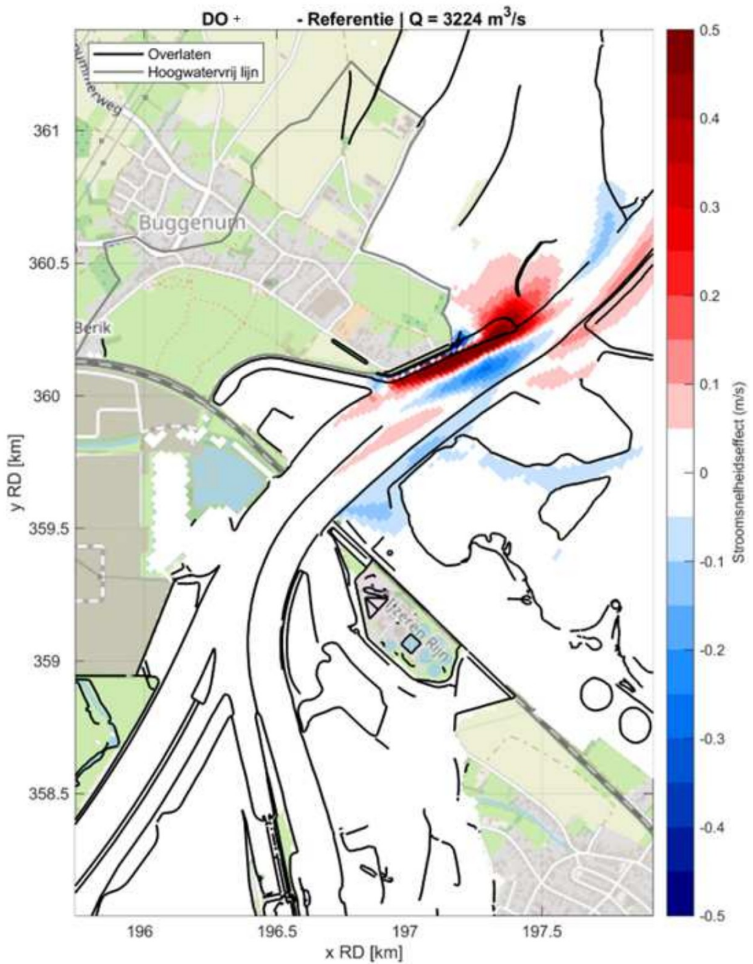
Fig. E.15: Stroomsnelheidseffect ten gevolge van het DO+ rondom de projectlocatie bij een afvoer van 3224 m 3 /s. Een rode kleur betekent een verhoging van de stroomsnelheid door het DO+.
