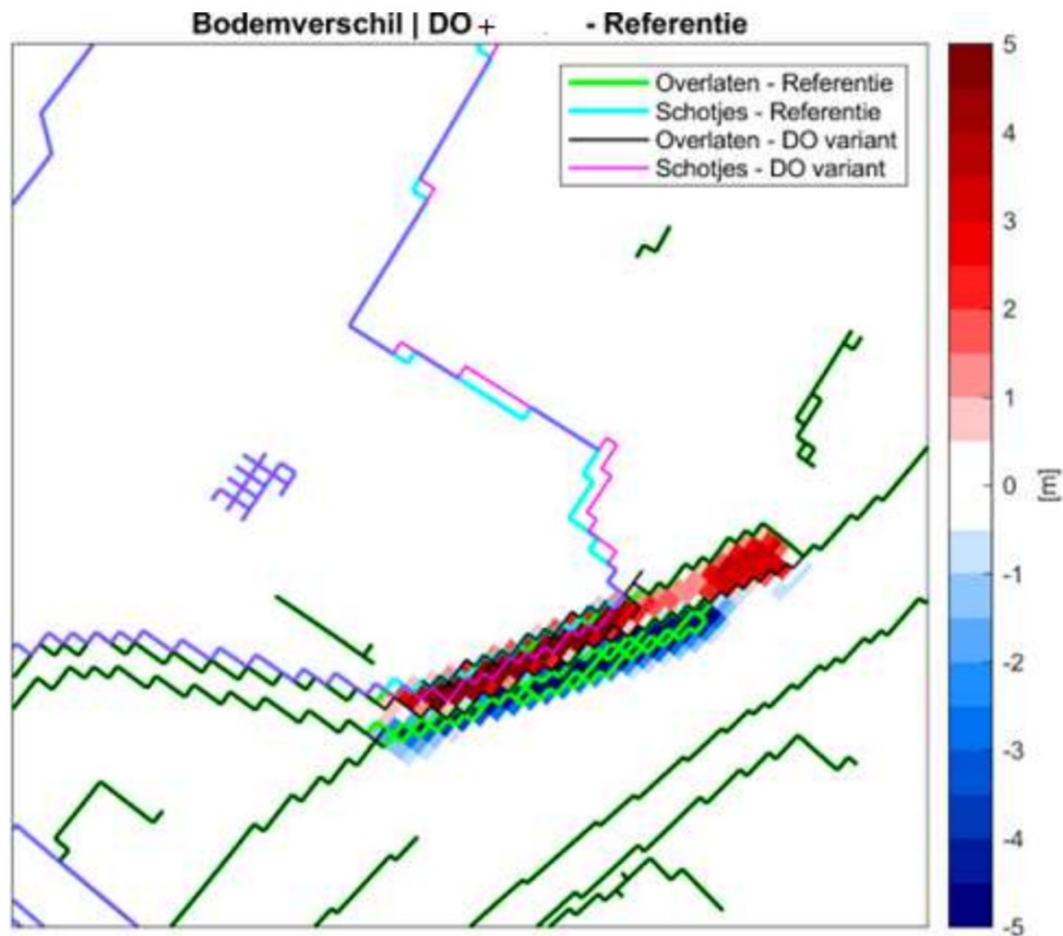
Figuur 3-3: Bodemligging in het Waqua model, met daarbij de overlaten en schotjes geplot. Het bovenste paneel weergeeft de referentiesituatie, het onderste paneel het DO+.
